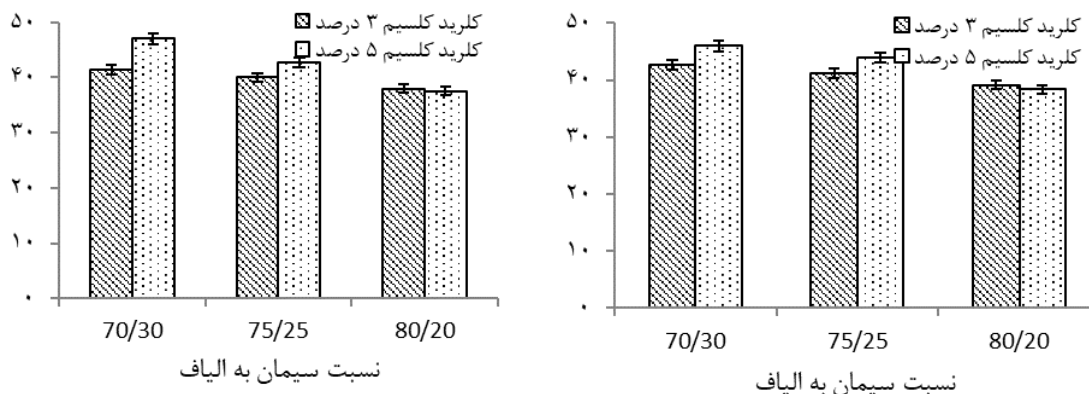
شکل ۱- اثر متقابل مقدار سیمان و کلرید کلسیم بر جذب آب تخته‌ها در ۲ و ۲۴ ساعت
