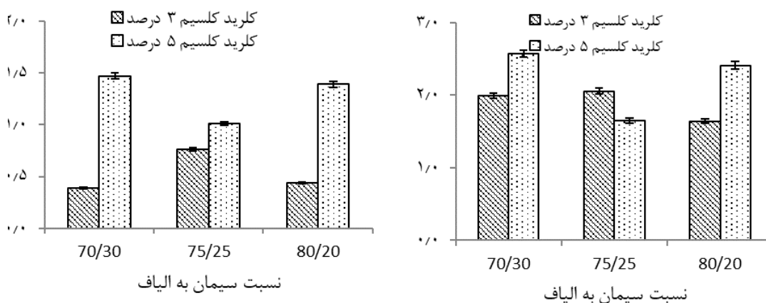
شکل ۲- اثر متقابل مقدار سیمان و کلرید کلسیم بر واكشیدگی ضخامت تخته‌ها در ۲ و ۲۴ ساعت
