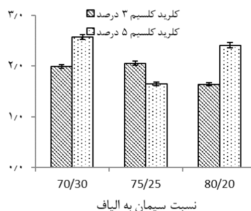
شکل ۲- اثر متقابل مقدار سیمان و کلرید کلسیم بر واكشیدگی ضخامت تخته‌ها در ۲ و ۲۴ ساعت
