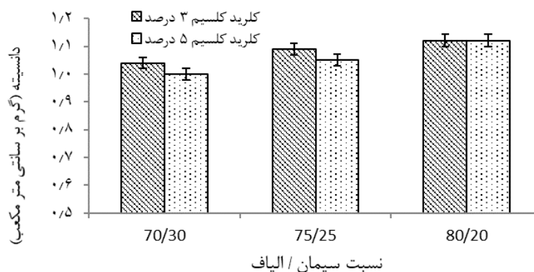
شکل ۳- اثر متقابل مقدار سیمان و کلیرد کلسیم بر دانسیته تخته‌ها
