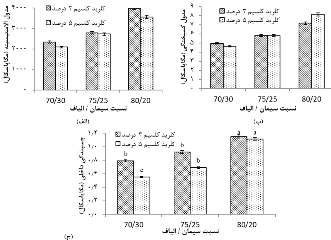
شکل ۴- اثر متقابل مقدار سیمان و کلرید کلسیم بر مدول الاستیسیته (الف)، مدول گسیختگی (ب) و چسبندگی داخلی (ج) تخته‌ها
