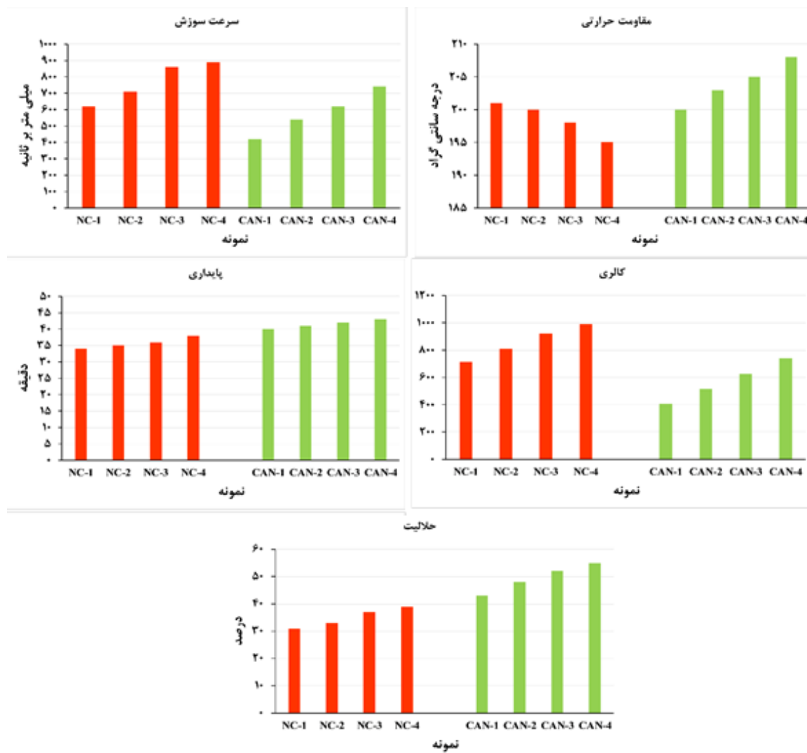
شکل ۳- مقایسه ویژگی‌های فیزیکی نمونه‌های تهیه شده از نیتروسولوز (NC) و نیتروسولوز استیله شده (CNA)
