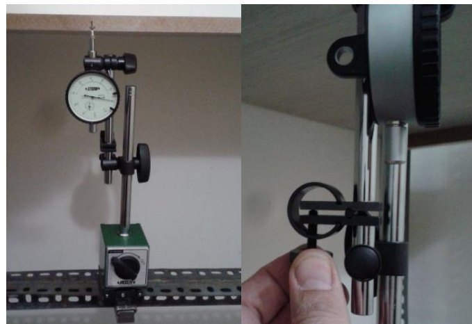
شکل ۲- خیز سنج مورد استفاده به همراه نحوه اندازه‌گیری خیز
