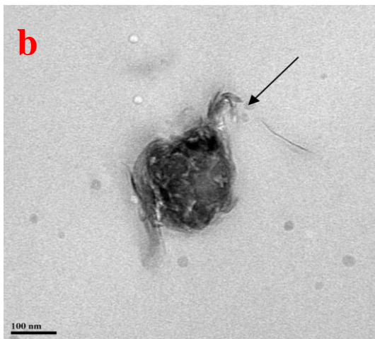
شکل ۲- میکروگراف میکروسکوپ الکترونی چندسازه آرد چوب- پلی پروپیلن (a) phc ۳ نانورس (b) phc ۵ نانورس
