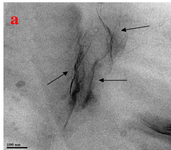
شکل ۲- میکروگراف میکروسکوپ الکترونی چندسازه آرد چوب- پلی پروپیلن (a) phc ۳ نانورس (b) phc ۵ نانورس
