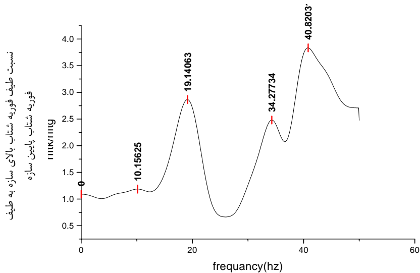
شکل ۷- فرکانس های نقاط اوج نمودار نسبت دامنه طیف فوری به شتاب بالای سازه به طیف فوری شتاب پایین سازه (rFFTk/rFFTg) در آزمون
