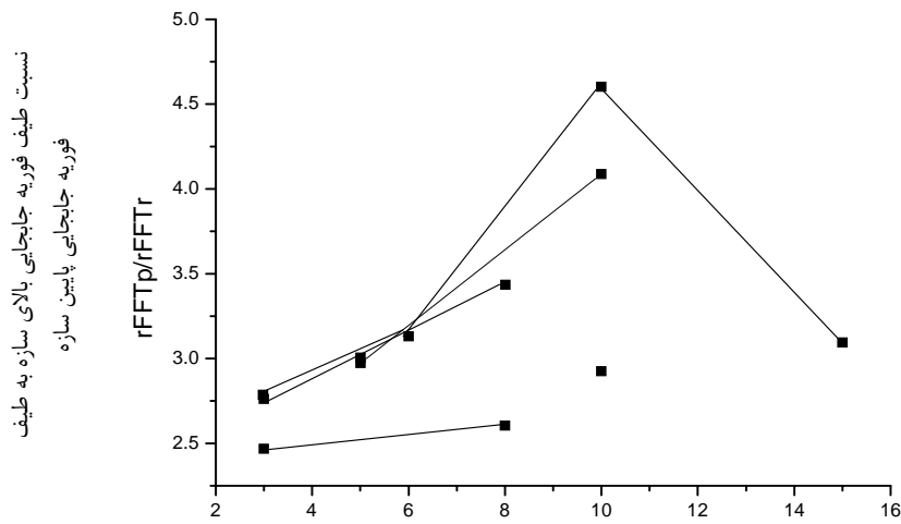
شکل ۶- نسبت طیف فوری به بیشینه جابجایی بالای سازه (rFFT p) به طیف فوری به بیشینه جابجایی پایین سازه (r FFT r) در برابر فرکانس برای آزمون های فرکانس سینوسی
