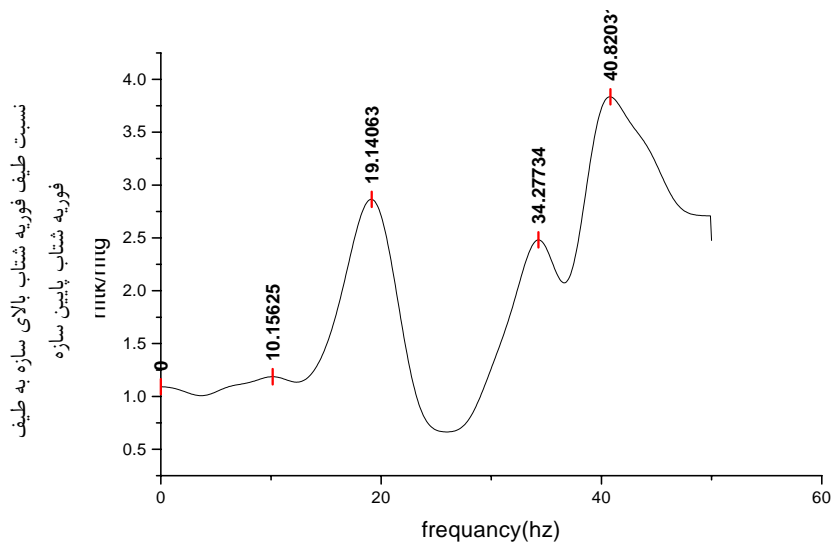
شکل ۷- فرکانس های نقاط اوج نمودار نسبت دامنه طیف فوری به شتاب بالای سازه به طیف فوری شتاب پایین سازه (FFTk/FFTg) در آزمون
