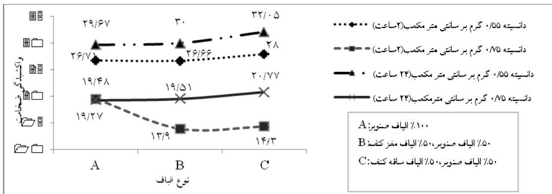
شکل ۴- مقایسه واكشیدگی ضخامت تخته‌های ساخته شده از ترکیب الیاف صنوبر- مغز کنف، صنوبر- ساقه کنف و صنوبر پس از ۲ و ۲۴ ساعت غوطه‌وری در آب
