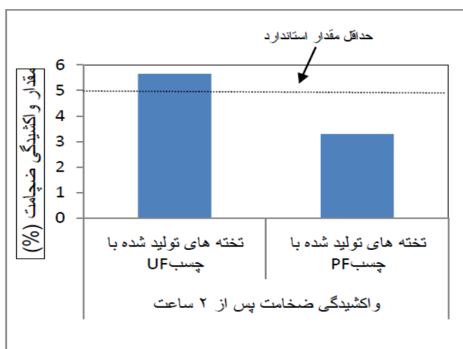
نمودار ۳- میزان واكشیدگی ضخامت پس از ۲ ساعت غوطه وری در آب
