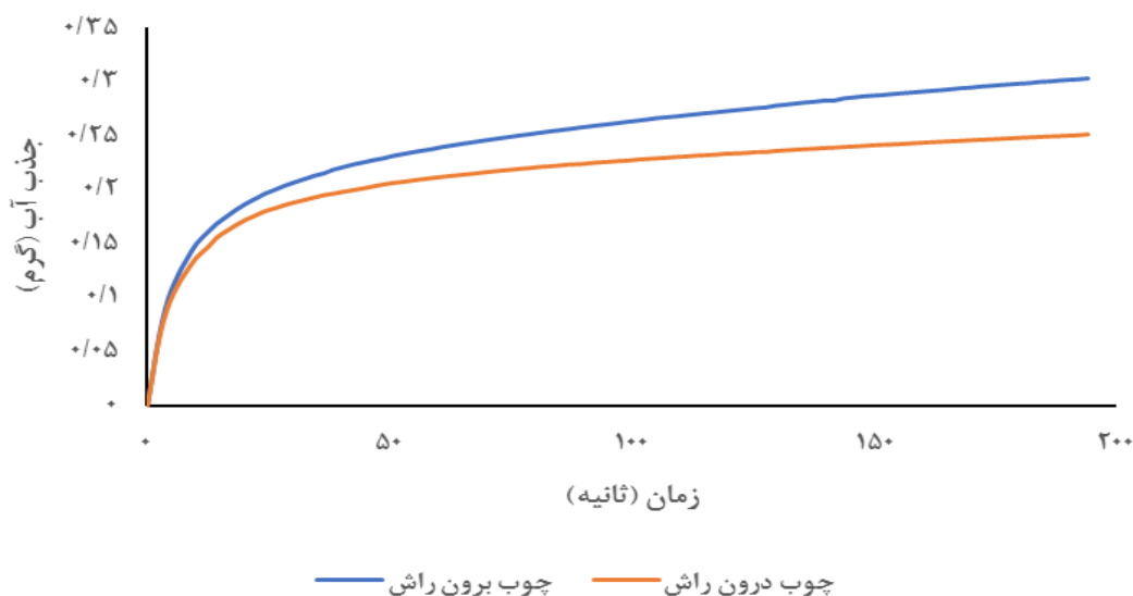
شکل ۱- نمودار جذب موئینه آب توسط تنسیومتر در مدت ۲۰۰ ثانیه
