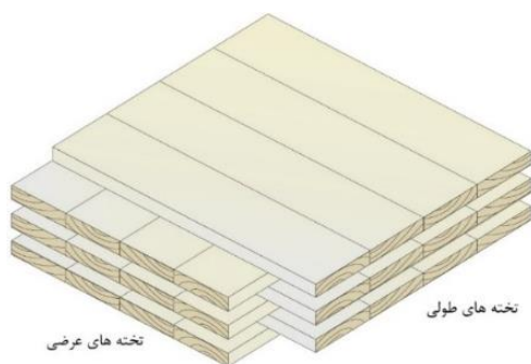
شکل ۱- نمایی از نحوه چیدمان لایه‌های CLT و محصول واقعی و کاربرد آن در ساختمان
