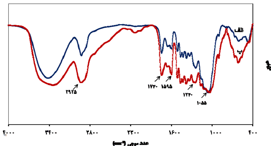
شکل ۳ - طیف‌سنجی مادون‌قرمز (FTIR). (الف) نمونه شاهد و (ب) نمونه تیمار شده در غلظت ۱۵ درصد
