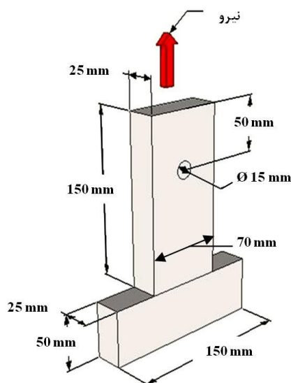
شکل ۲- نمایشی از نمونه آزمون توان نگهداری
