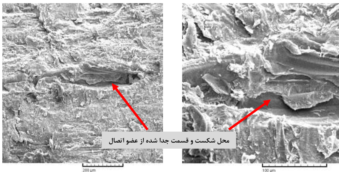
شکل ۵- تصویر میکروسکوپ الکترونی روبشی از محل شکست عضو و دوپل در اتصال جوشکاری شده
