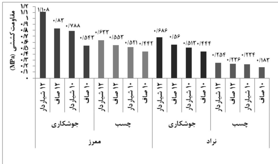
شکل ۱- مقاومت کششی در اتصال‌های دوبل ساخته شده به دو روش جوشکاری و چسب PVA
