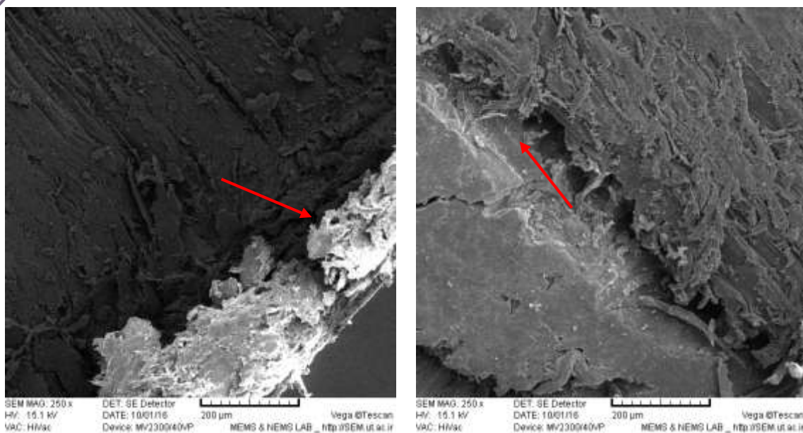
شکل ۲- ریزنگار میکروسکوپ الکترونی تهیه شده از ناحیه اتصال با جوشکاری (فلش قرمز) که درگیر شدن سلول‌های چوبی (فیبر تصویر راست و تراکئیدها تصویر چپ) را طی جوشکاری نشان می‌دهد.
