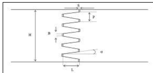
شکل ۱- ژئومتری اتصال انگشتی مورد استفاده در تحقیق
