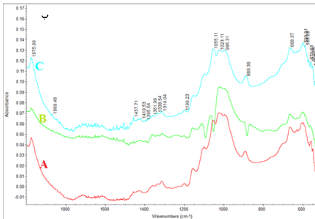
شکل ۲- الف، A: کاغذ مرکب مازو، B: مرکب مازو تیمار شده با تیوفانات متیل، B: مرکب مازو تیمار شده با تیوفانات متیل، C: مرکب مازو تیمار شده با تیوفانات متیل، B: مرکب مازو تیمار شده با تیوفانات متیل، B: مرکب مازو تیمار شده با تیوفانات متیل، C: کهنه‌سازی شده در ۶ روز، C: مرکب مازو تیمار شده و کهنه‌سازی شده در ۱۲ روز.
