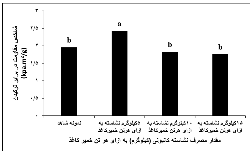
شکل ۴- اثر نشاسته کاتیونی در تیمارهای مختلف بر روی شاخص مقاومت در برابر ترک‌کین کاغذهای دست‌ساز
