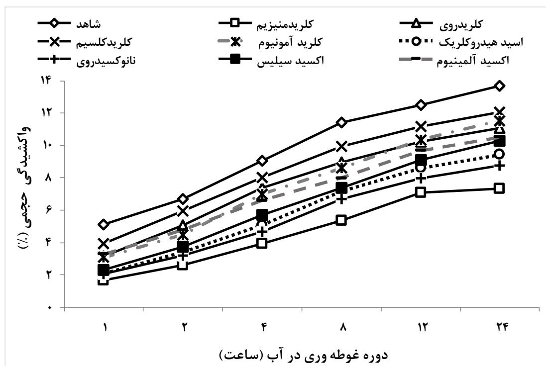
شکل ۴- اختلاف واکنش حجمی بین کاتالیزورهای گلو تار آلدئید
