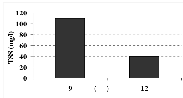
شکل ۷- اثر مستقل ولتاژ روی کاهش TSS پساب
