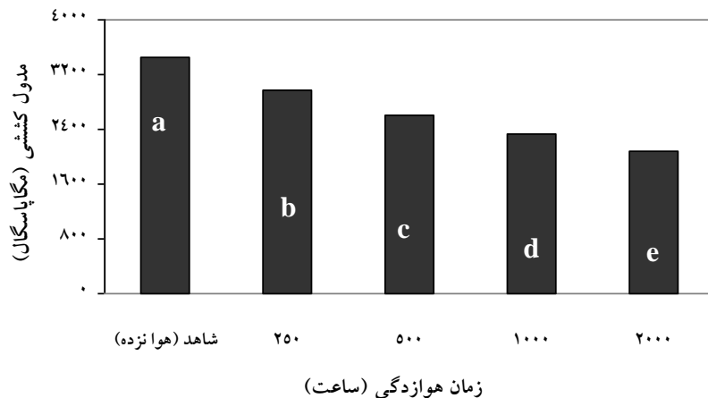
شکل ۴- تأثیر زمان هوازگی بر مدول کششی چندسازه آرد چوب- پلی اتیلن سنگین
